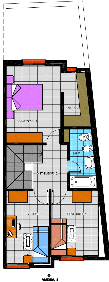
PLANTA PRIMERA
