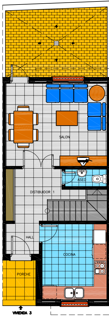
PLANTA BAJA
