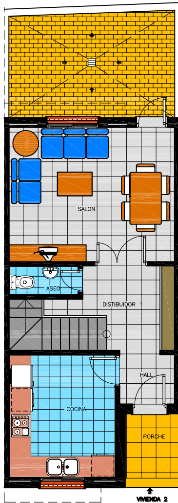
PLANTA BAJA
