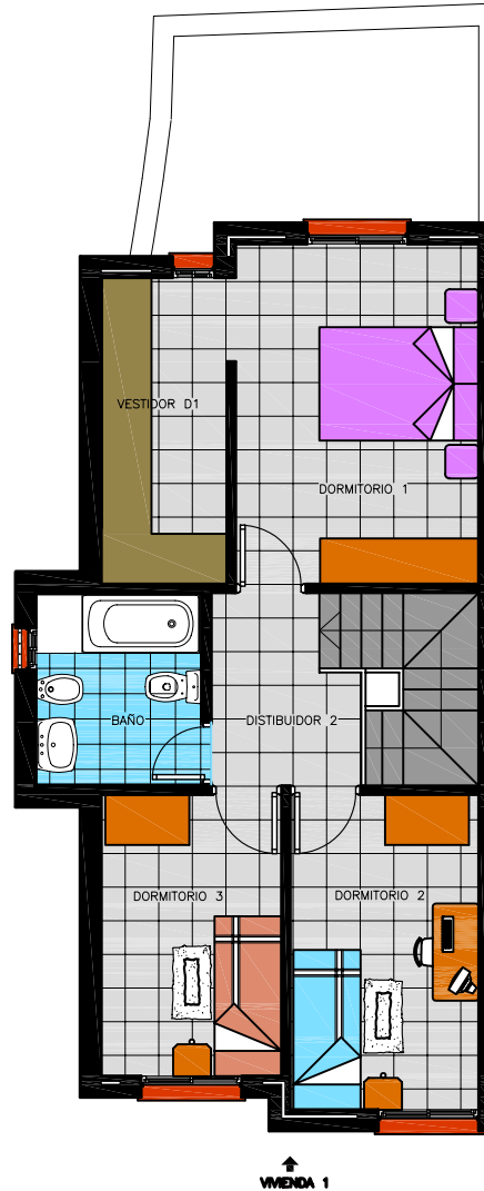
PLANTA PRIMERA
